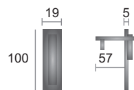
C1165 Pocket Door Edge Pull
